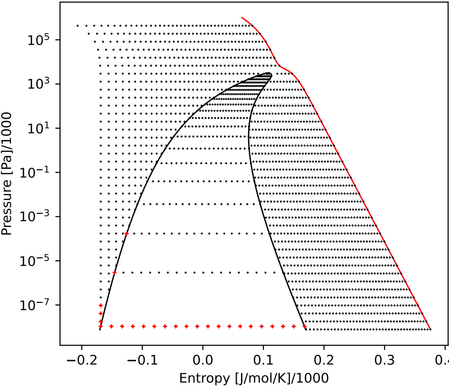
DmolarP
