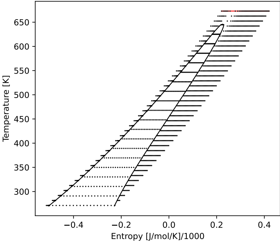
DmolarHmolar
