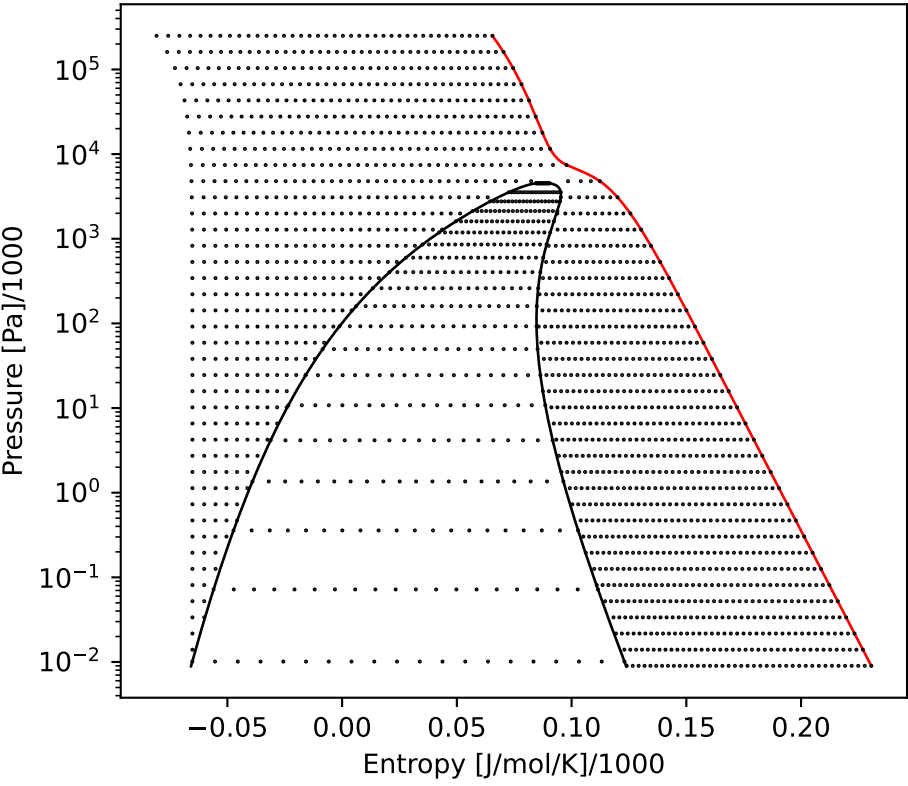
DmolarP
