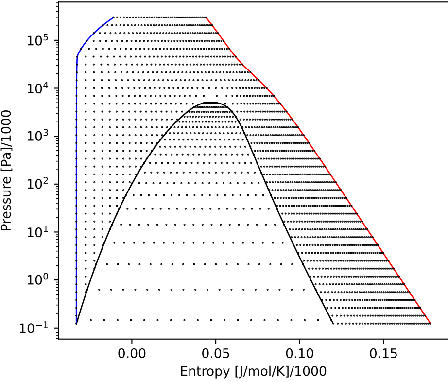
DmolarP
